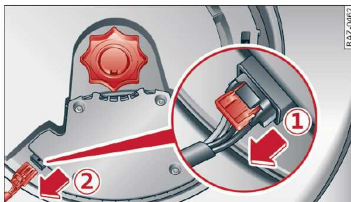
Fig. 161 Spare tire well: subwoofer
